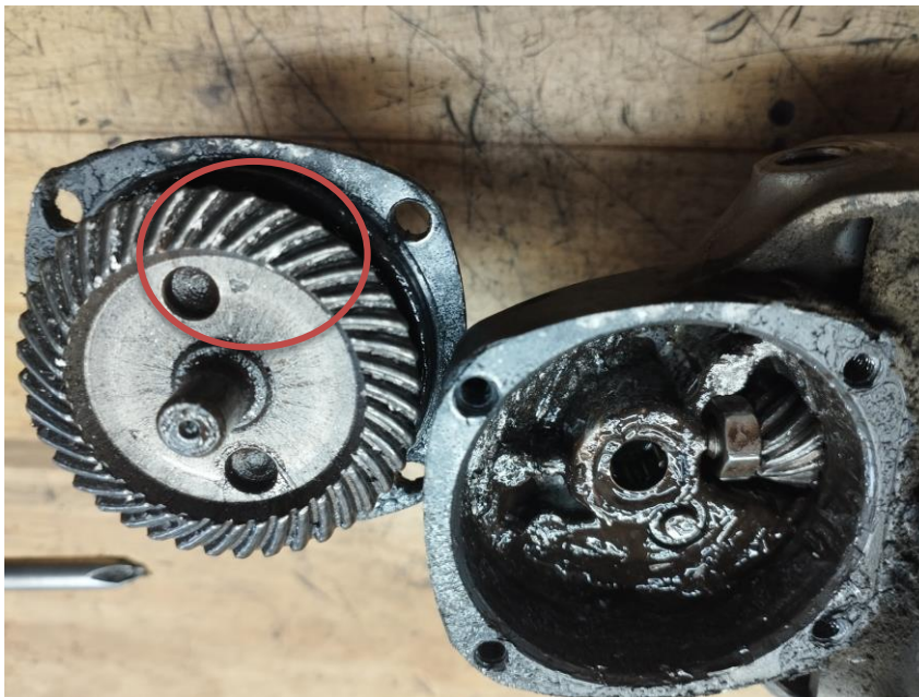
Obr.2 Opatrebenie ozubených prevodov
