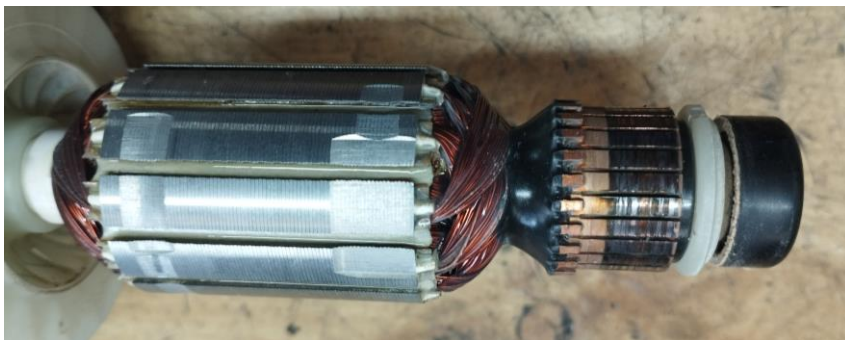
Obr.2 Rotor BX800
