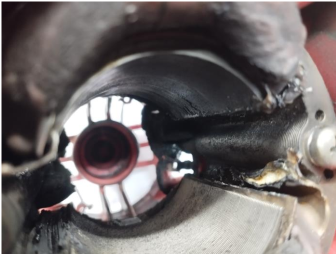
Obr.2 Poškodenie statora
