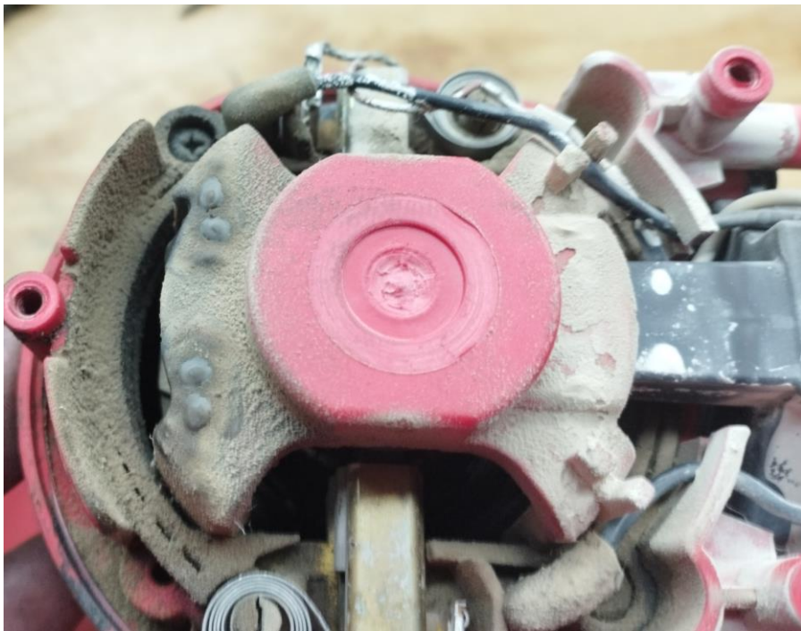
Obr.2 Zanesenie držiaka kief nečistotami
