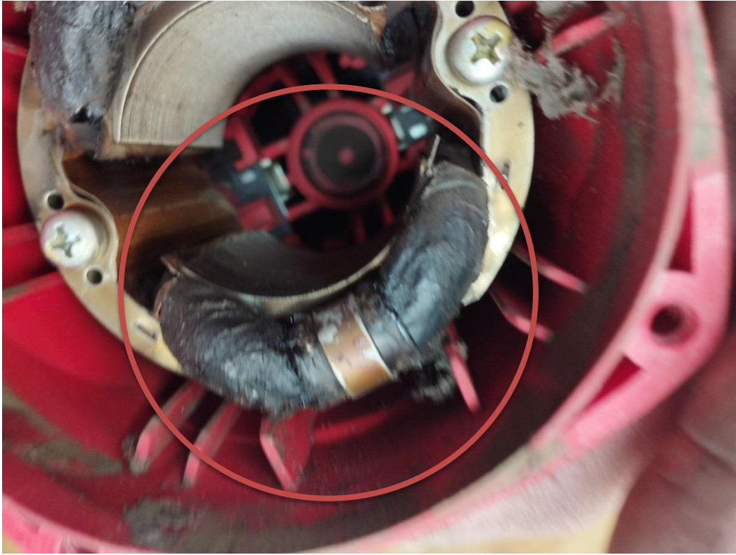
Obr.1 Poškodenie statora
