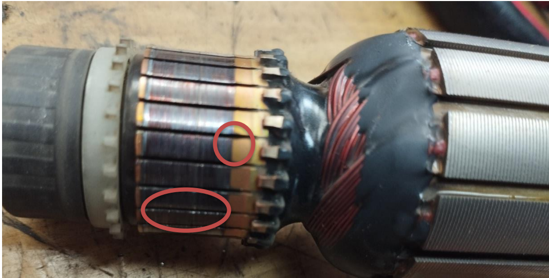
Obr.2 Poškodenie komutátora rotora
