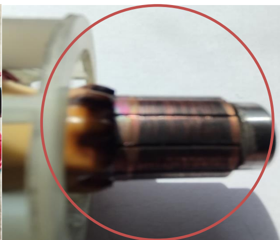
Obr.2 Poškodenie komutátora rotora
