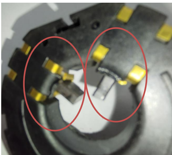
Obr.3 Poškodenie držiaka kief
