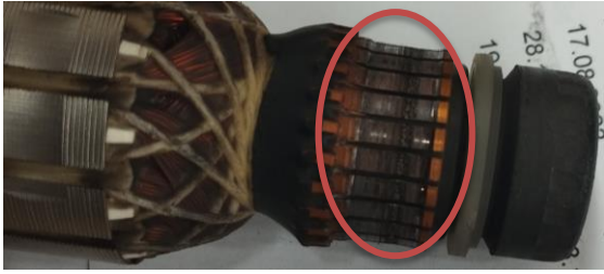
Obr.1 Poškodenie komutátora
