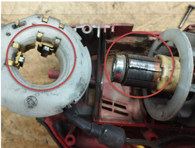
Obr.2 Poškodenie komutátora, opotrebenie kief
